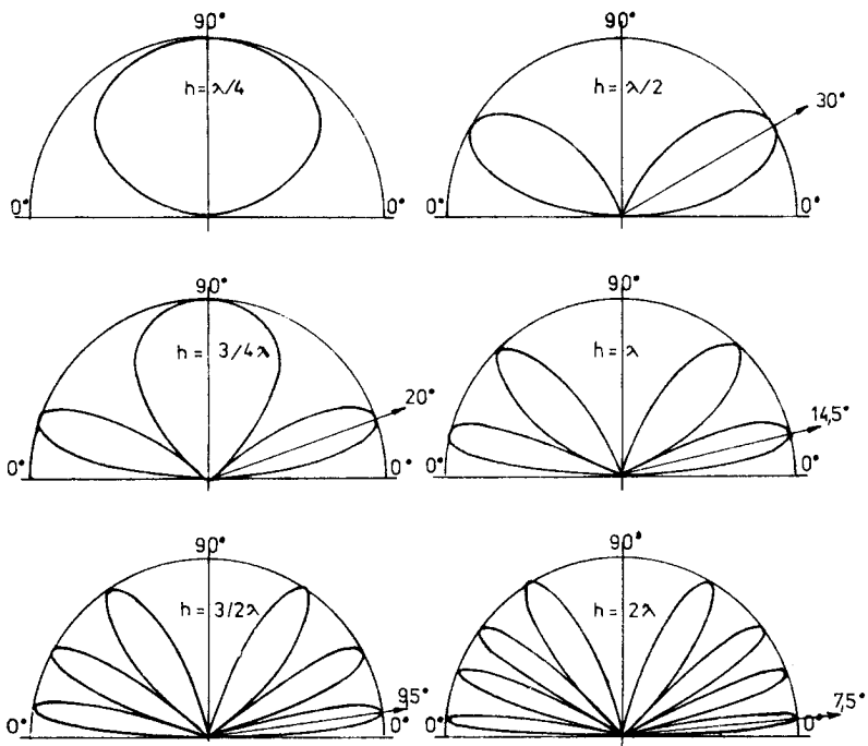
Obr.14. Vertikální vyzářovací diagramy horizontálního půlvlnného dipólu v závislosti na výšce nad zemí
