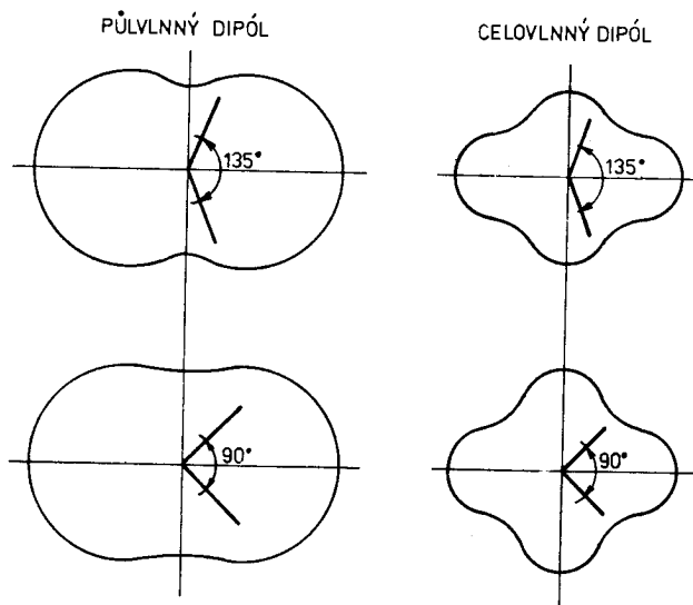
Obr.42. Vyzařovací diagramy "zahnutých" dipólů
