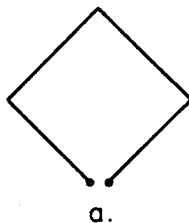
Obr.56. Celovlnná smyčka a/ horizontální polarizace b/ vertikální polarizace
