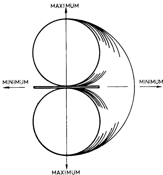
Obr.9. Prostrový vyzářovací diagram půlvlnného dipólu ve volném prostoru
