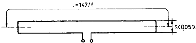
Obr.37. Skládáný dipól
