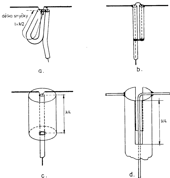
Obr.31. Různé způsoby symetrizace souosého vedení
