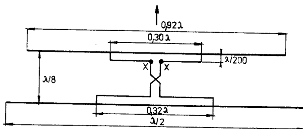
Obr.52. Směrová anténa HB9CV
