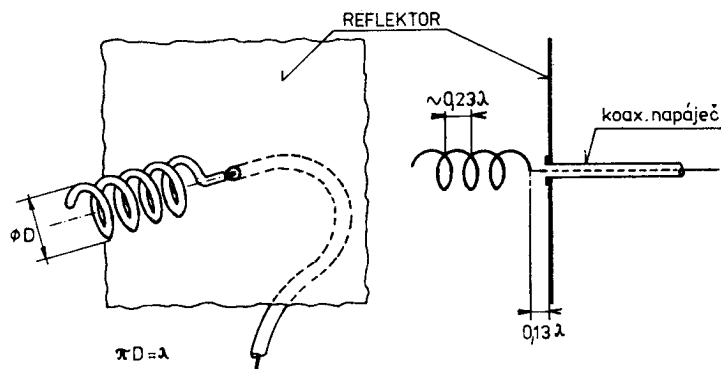
Obr.71. Šroubovicová anténa
