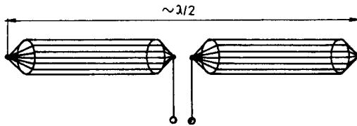
Obr.36. Širokopásmový dipól
