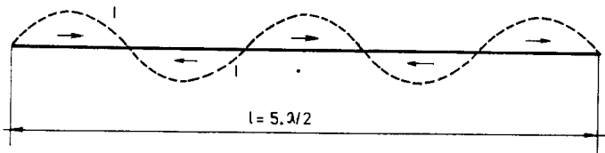
Obr.44. Rozložení okamžitých proudů na dlouhém zářiči
