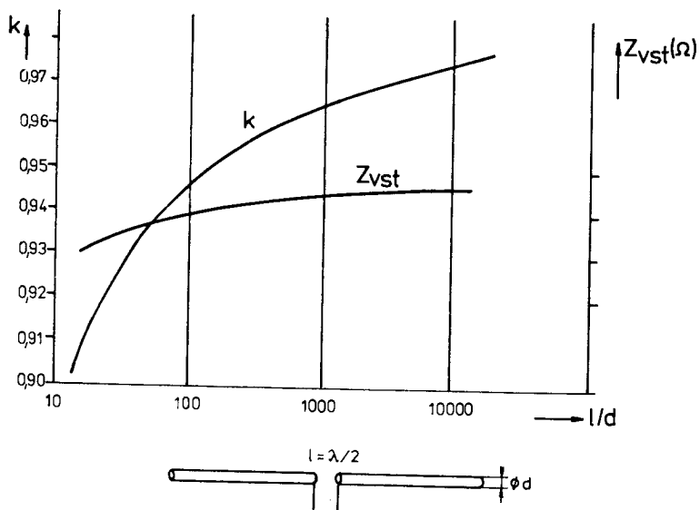
Obr.7. Závislost činitele zkrácení a vstupní impedance půlvlnného dipólu na poměr l/d
