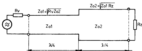
Obr.22. Dvojstupňový čtvrtvlnný transformátor pro větší transformační poměry R_z/R_v
