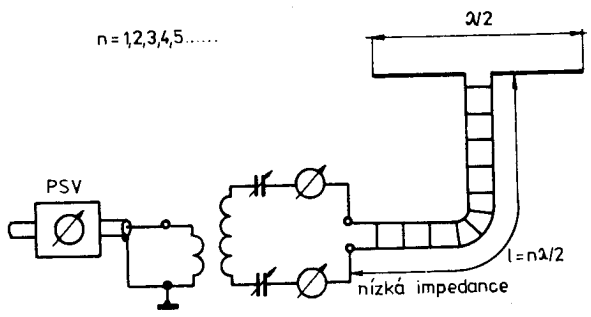
Obr.35. Vazební obvody pro laděné napáječe
