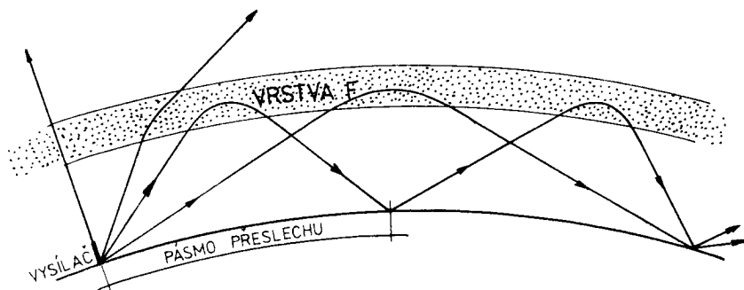
Obr.6. Šíření ionosférické vlny a význam elevačního úhlu
