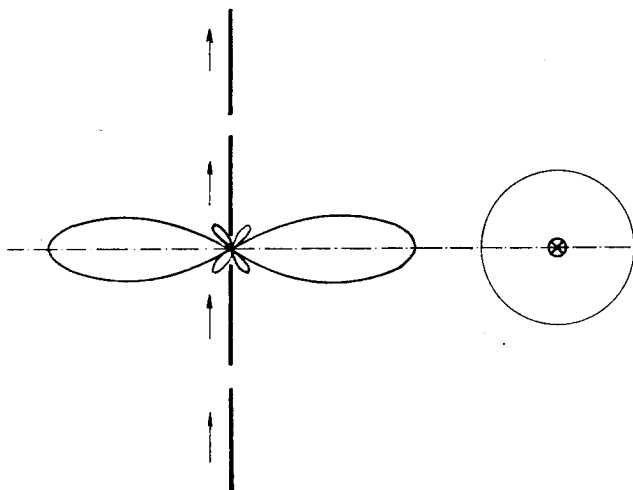
Obr.47. Vyzářování řadové soustavy
