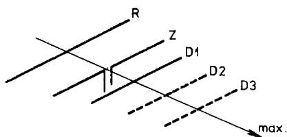
Obr.54. Víceprvková anténa Yagi R ... reflektor Z ... zářič D ... direktory
