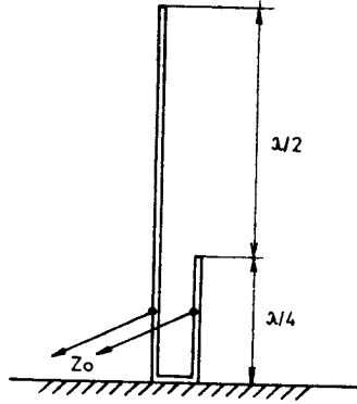
Obr. 63. Anténa "J"
