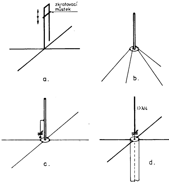
Obr.62. Různé způsoby přizpůsobení vstupní impedance antény GP
