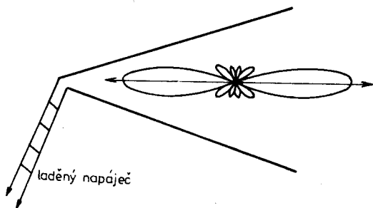
Obr.46. Směrová anténa "Y"
