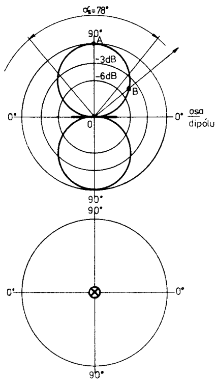
Obr.10. Vyzařovací diagram půlvlnného dipólu v rovině zářiče a v rovině kolmé
