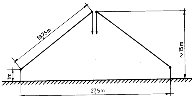
Obr.43. Anténa "obrácené V"
