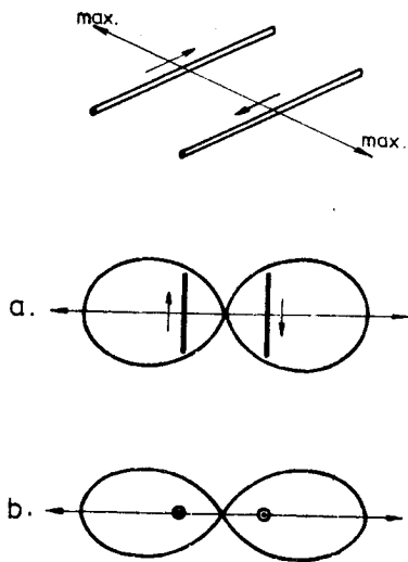
Obr.51. Koncová soustava
