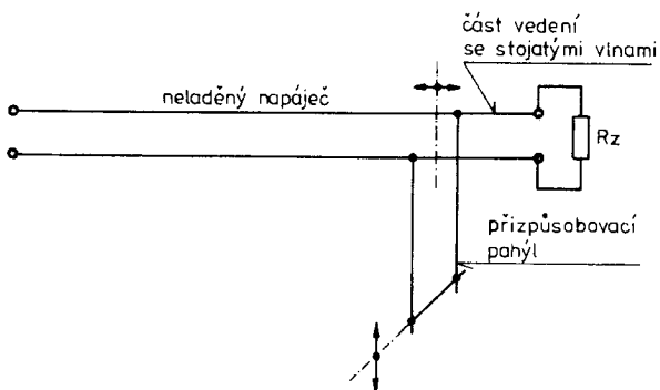
Obr.26. Přípůsobení impedancí pahýlovým vedením
