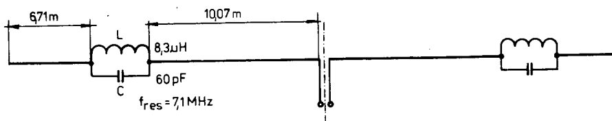
Obr.41. Vícepásmový dipól podle W3DZZ
