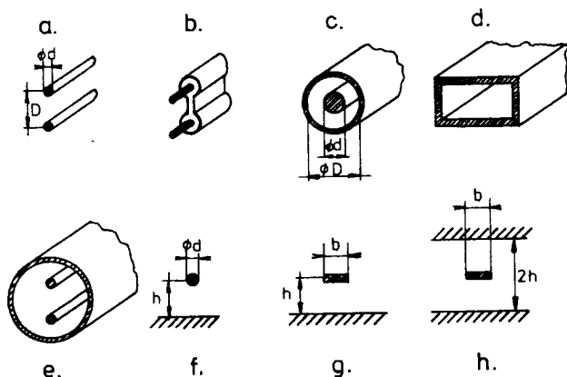
Obr.16. Nejčastěji používané typy vř vedení
