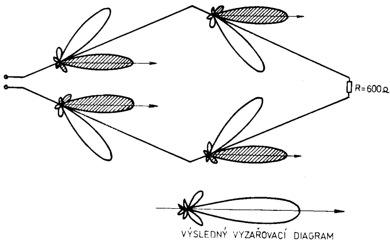
Obr.12. Kosočtverečná anténa
