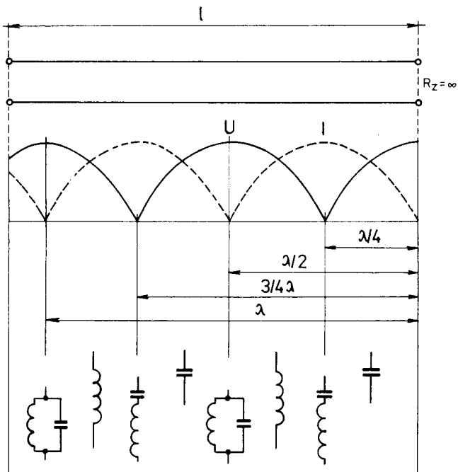
Obr.20. Vlastnosti vedení naprázdno
