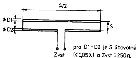
Obr.29. Skládáný dipól
