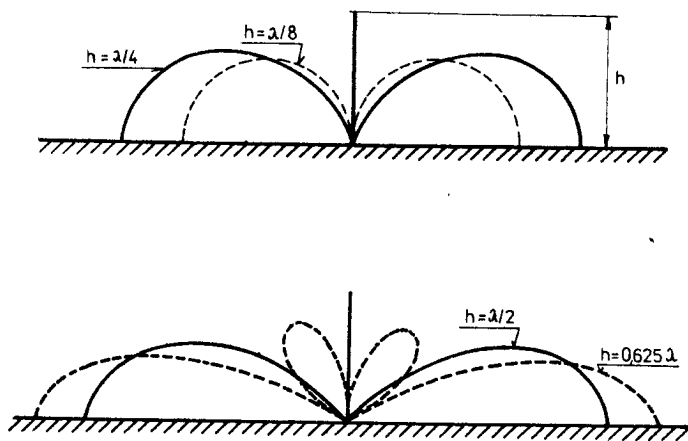
Obr.59. Vertikální vyzařovací diagramy různé vysokých vertikálních zářičů
