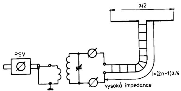
Obr.34. Typické vazební obvody pro VKV vysílače
