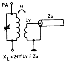
Obr.34. Typické vazební obvody pro VKV vysílače
