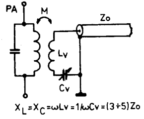
Obr.34. Typické vazební obvody pro VKV vysílače
