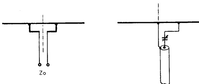
Obr.28. Bočníkové přizpůsobení a/ přizpůsobení "T" b/ přizpůsobení "gama"
