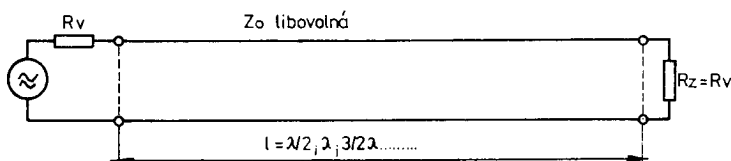
Obr.23. Transformace impedancí 1:1 půlvlnným vedením
