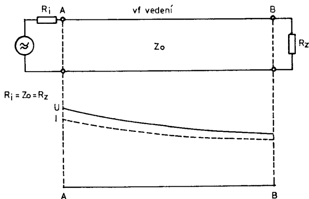
Obr.17. Přizpůsobené vedení
