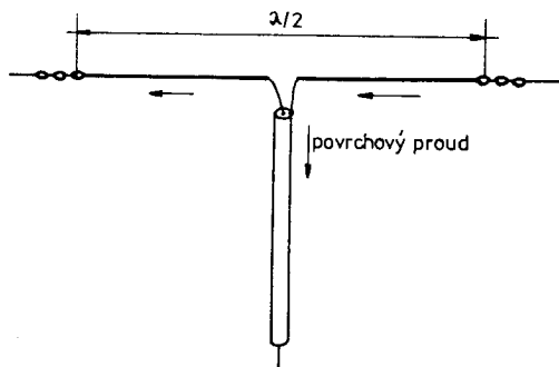
Obr.30. Chybné napájení symetrického zariadení nesymetrickým napáječem
