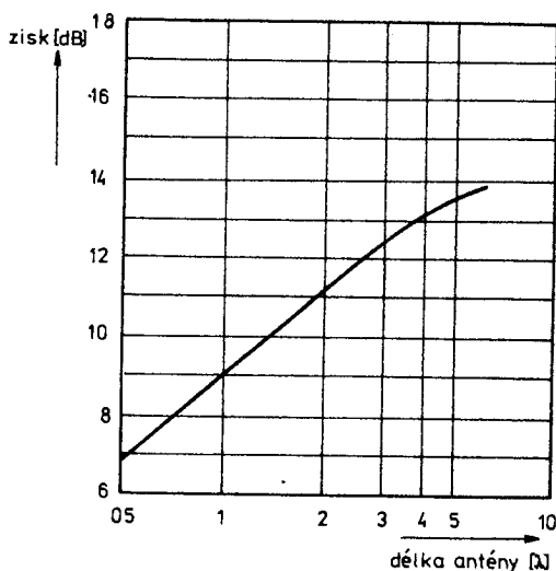
Obr. 65. Závislost zisku antény Yagi /proti půlvlnnému dipólu/ na její délce
