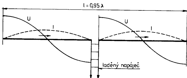
Obr.39. Celovlnný dipól s vyznačeným průběhem proudového a napětového obložení
