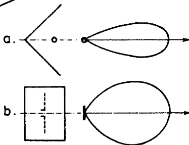
Obr.69. Úhlový reflektor
